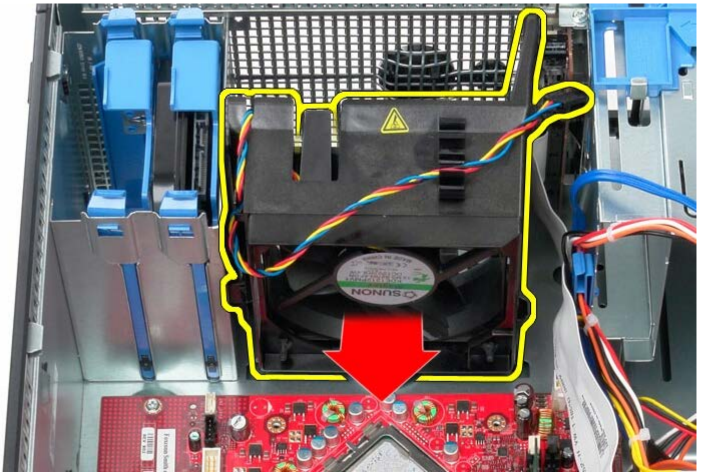
1 11 從電腦卸下處理器風扇。
