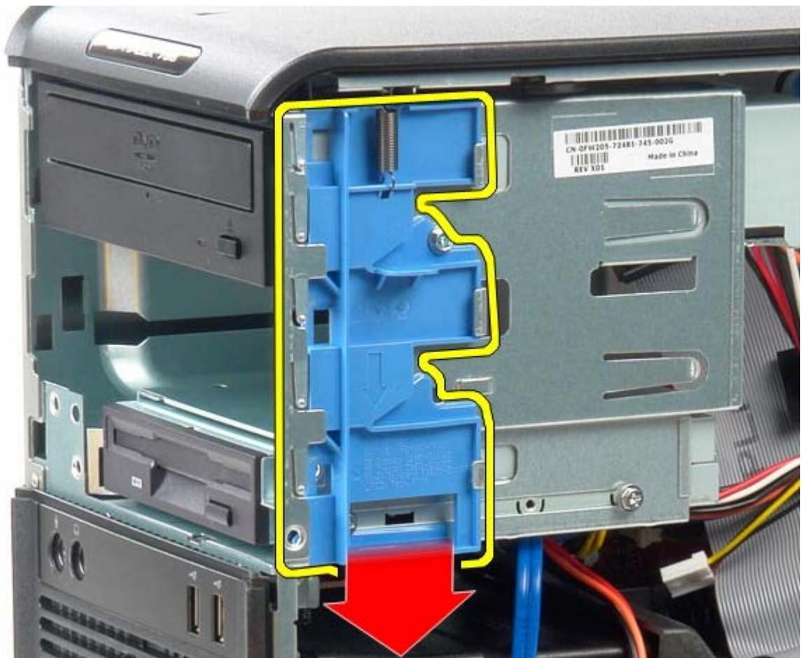
1 11 朝系統底座方向推動光碟機釋放門鎖並按住。
