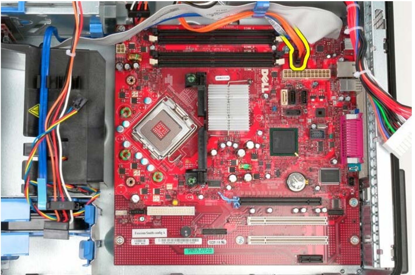
1 11 將光碟機資料纜線擺在一旁。
