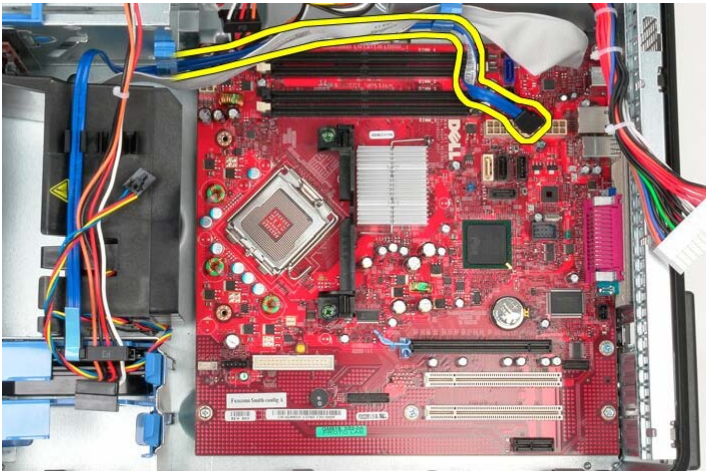
11 11 從主機板拔下 IO 面板資料纜線。
