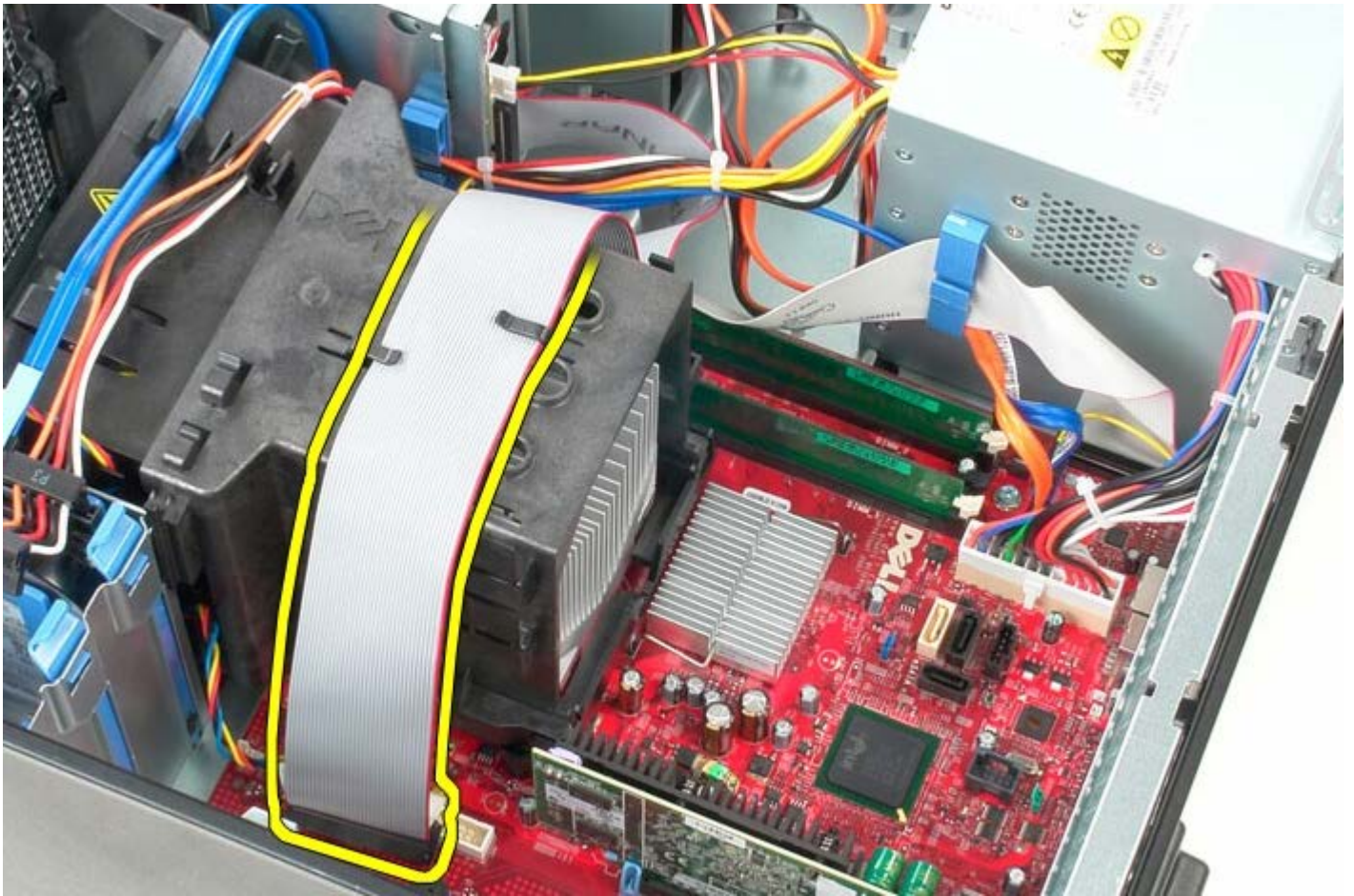
1 11 鬆開將散熱器固定至主機板的兩顆緊固螺絲。
