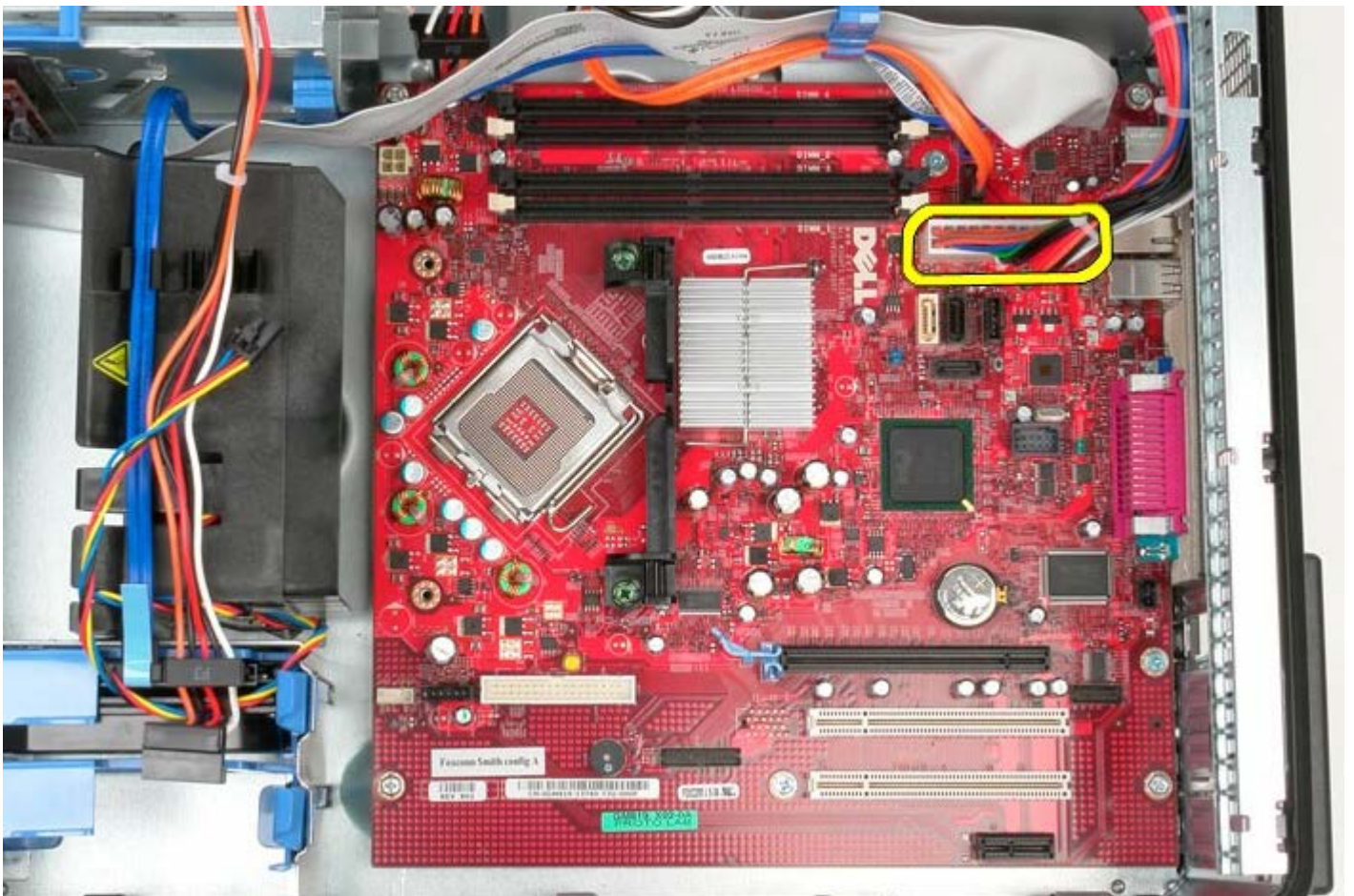
1 11 從主機板拔下光碟機資料纜線。
