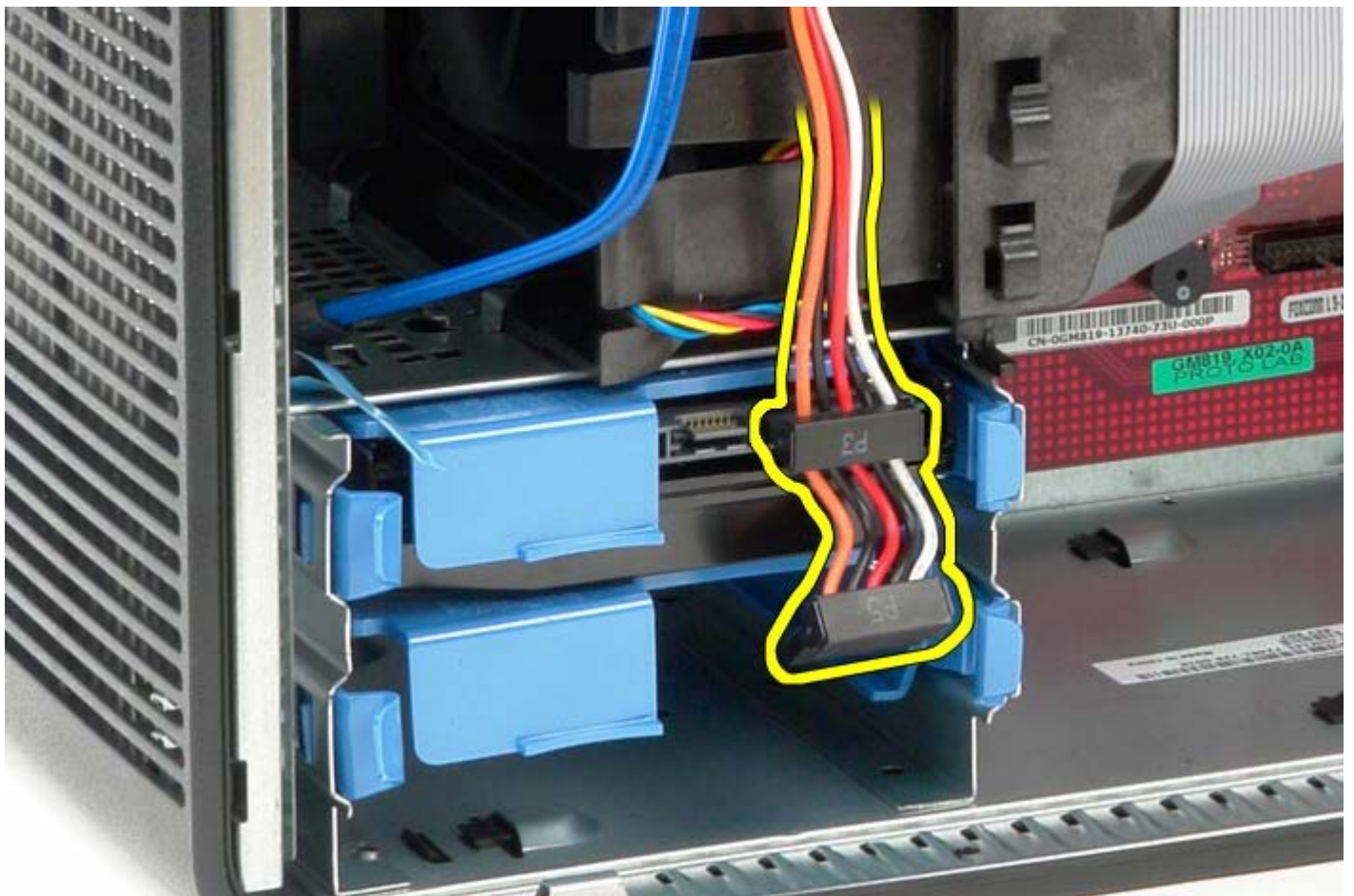
1 11 向內按壓硬碟機兩側的藍色釋放彈片。
