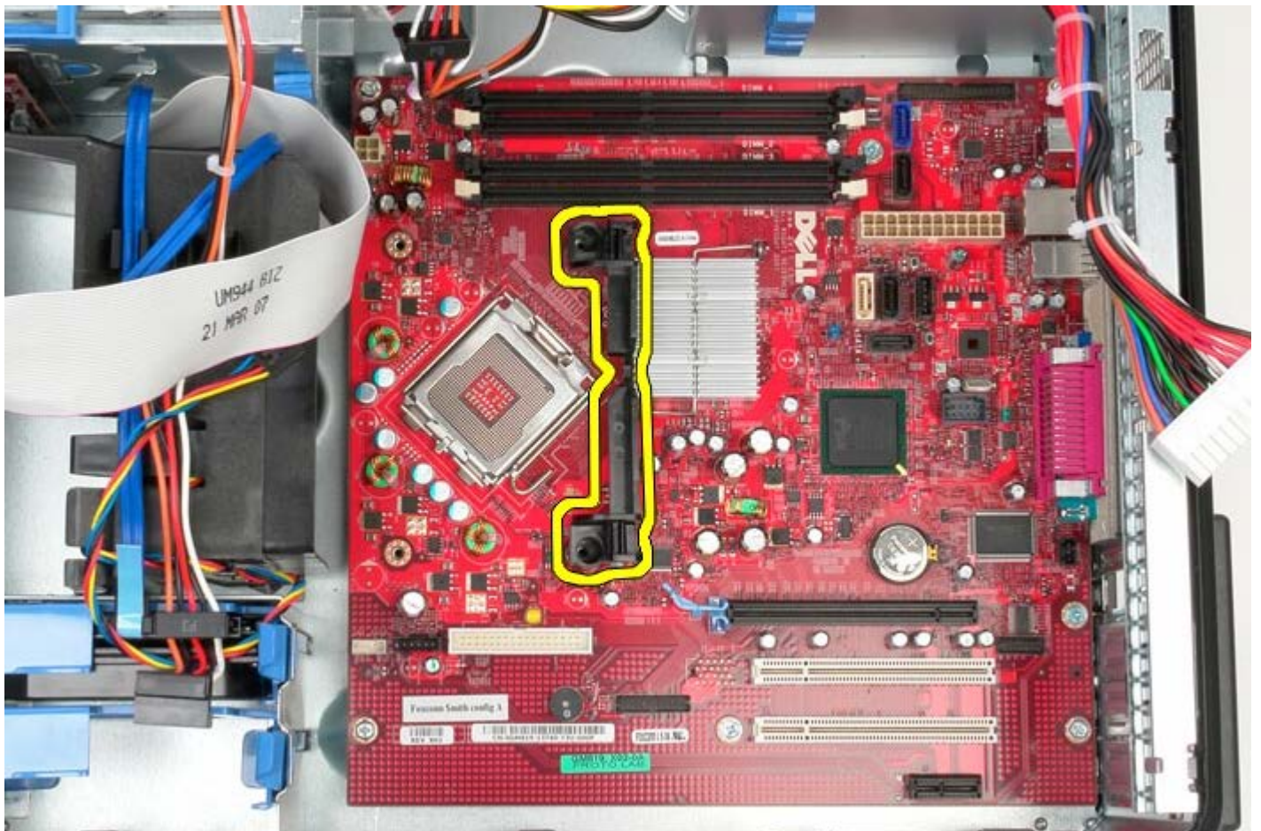
1 1 11 卸下將主機板固定到機箱的七顆螺絲。
