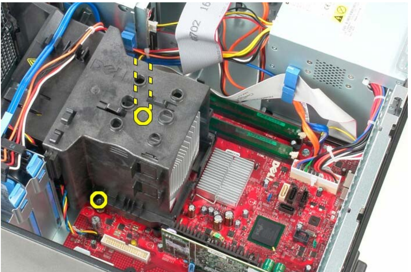
1 11 朝電腦背面轉動散熱器。
