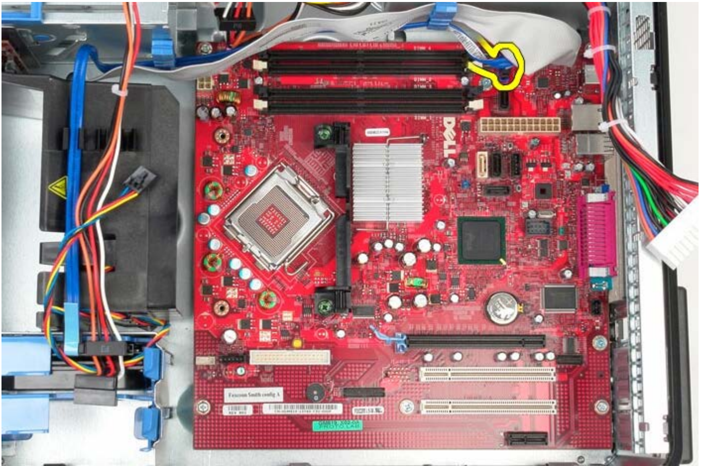
11 11 將硬碟機資料纜線擺在一旁。
