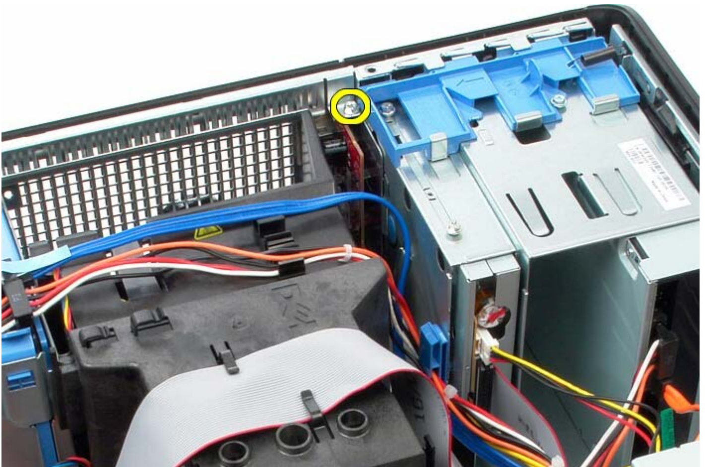
1 11 按壓固定門鎖，鬆開 IO 面板。
