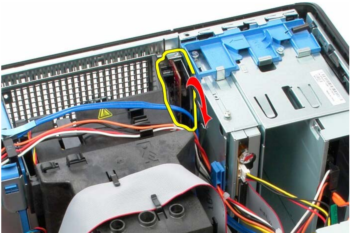
1 11 將 IO 面板從插槽提起取出。
