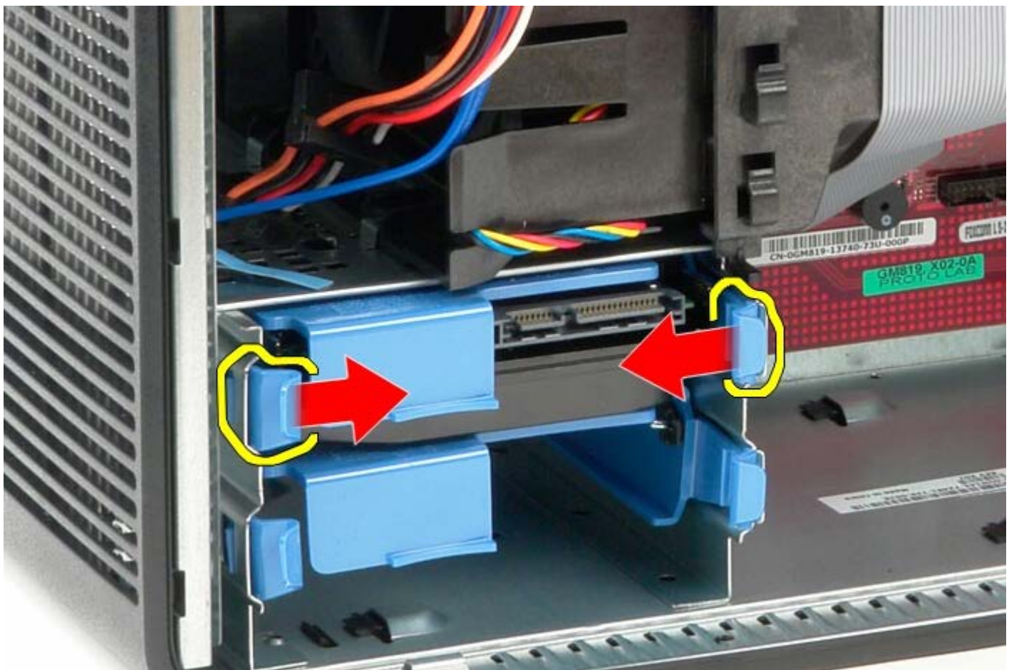
1 11 將硬碟機推出電腦。
