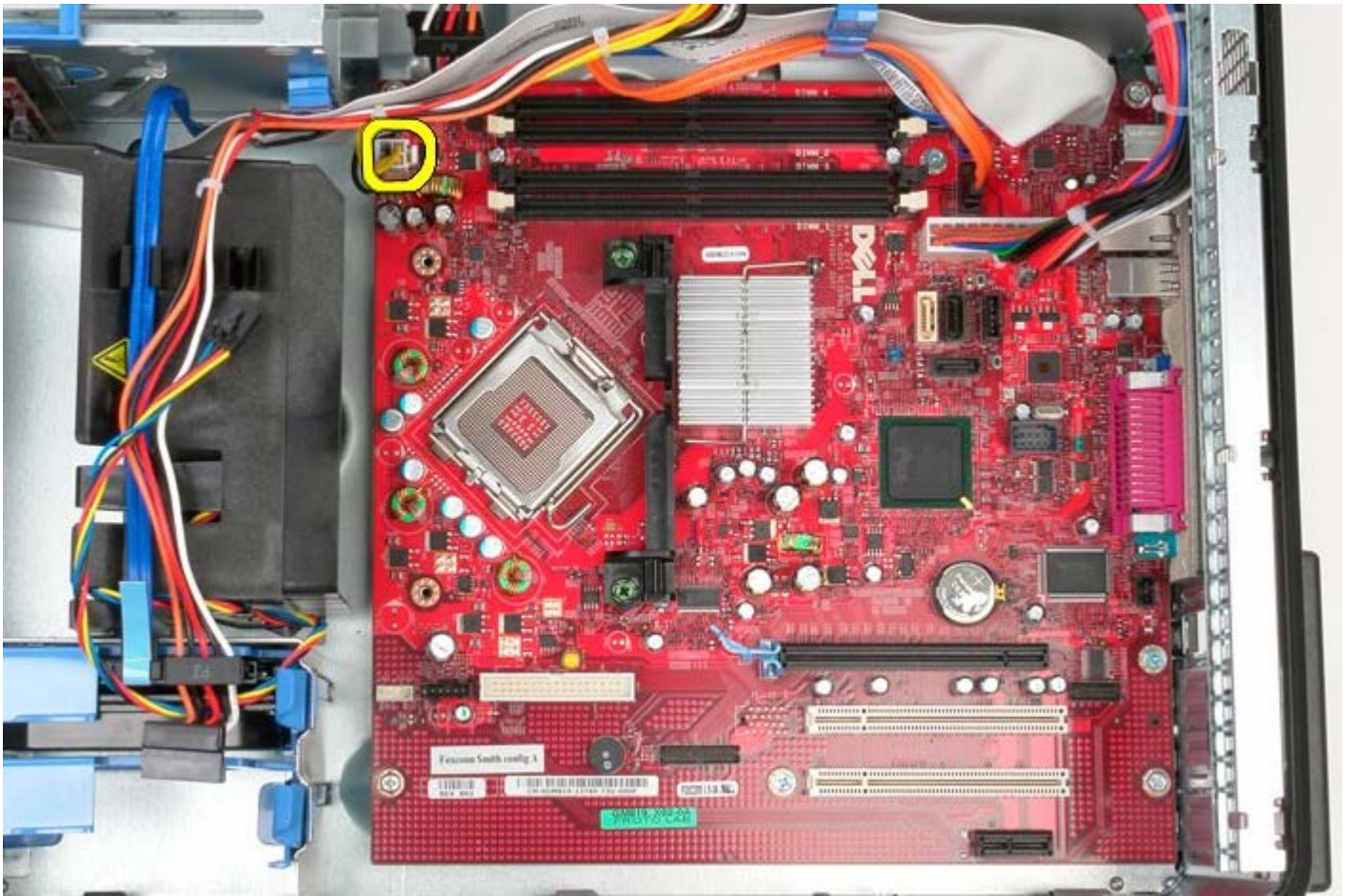
1 11 拔下主要的主機板電源線。
